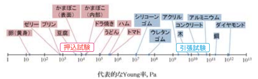
図3. あらゆる素材を、共通の指標(弾性係数)で評価可能とする計測法
