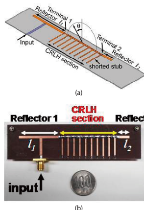
図2 0次共振器の構造 (a) 概略図 (b) 写真
