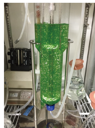
固定化エアリフトバイオリアクターによる遺伝子組み換え藍藻を用いたバイオアルコール生産
