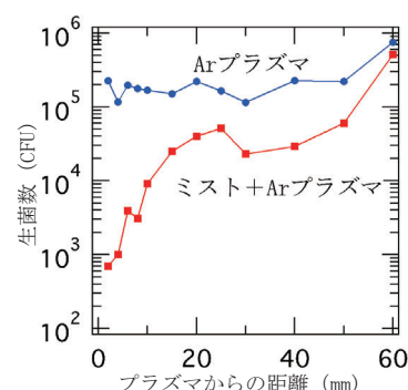
図2. ミストプラズマの殺菌効果
