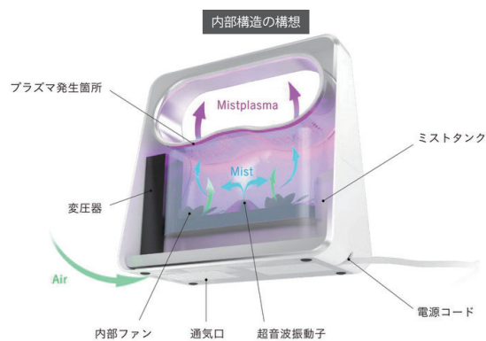
図4. ハンドサニタイザーの内部構造
