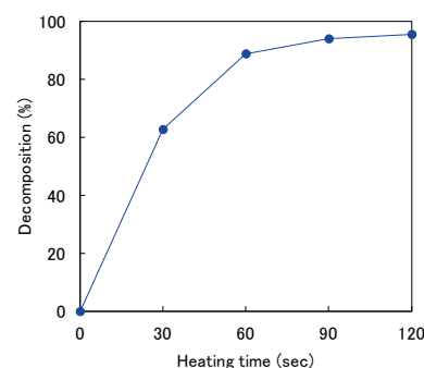
Fig.2 ホウフッ化物の分解に及ぼすマイクロ波加熱の効果 [BF 4 ]= 40ppm, [Al 3+ ]= 25ppm
