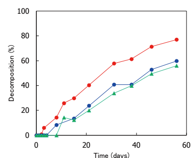
Fig. 1 ホウフッ化物の分解に及ぼすpHの影響 [BF 4 ]=40ppm, 25°C ● pH 3, ● pH 4, ▲ pH 5
