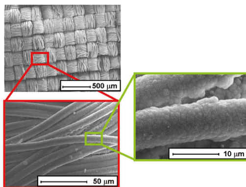
PET布帛より作製した高い空隙率と大きな比表面積を有するヒドロキシアパタイトとのハイブリッド繊維材料のSEM像
