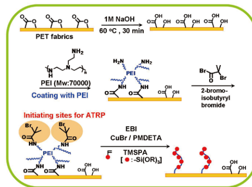
多段階の表面修飾反応からなるPET繊維／ヒドロキシアパタイトハイブリッドの作製プロセス
