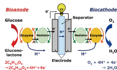
バイオ燃料電池の発電原理
