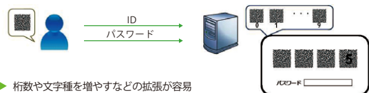
VSSSを用いたワンタイムパスワード認証の流れ
