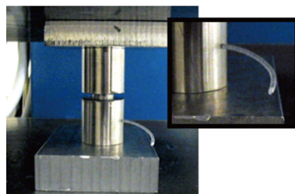
図1 生分解性バロプラスチックの室温成形の模様
