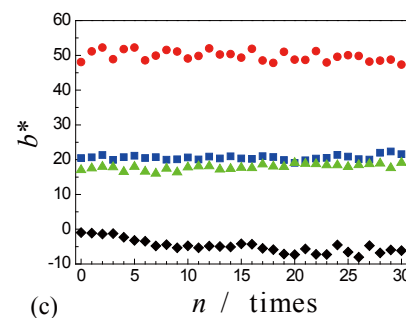
図3 カテキノン(●)、カテキノン+赤キャベツ色素混合系(▲)、PAP+5AOC(■)、酸性染料(◆)でそれぞれ染色した毛髪への洗髪回数 n に対する明度 ( L^* 、(a))、赤-緑色度 ( a^* 、(b))、黄-青色度 ( b^* 、(c)) の変化。
