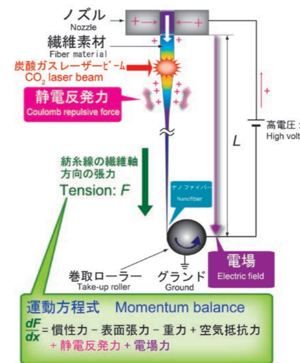
レーザーエレクトロスピニングプロセスの概念図
