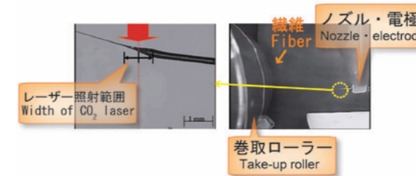
レーザーエレクトロスピニング (LES) の様子
