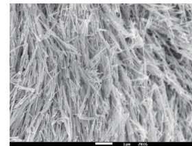
図4 メソ孔をテンプレートにナノ成形した例。スケールバーは1 \mu\text{m} 。
