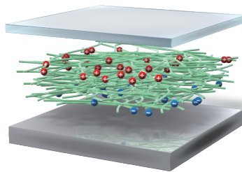
図2 不織布の疑似正圧電特性のモデル 不織布の内部で正電荷と負電荷が偏在しており、分極のような電荷の偏りが発生していると考えられる。
