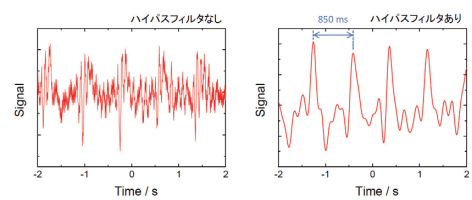
図3 心拍検出センサの検出結果 一次的に検出された信号を処理することで、心拍を算出することが可能(左・右グラフ)。
