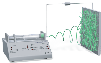
図1 電界紡糸法と不織布 基板とシリンジの間に高い電圧ををかけ、シリンジからポリマー溶液が放出され、基板に到達する前に有機溶剤が蒸発し、基板にはファイバーとして付着する。最終的にランダムメッシュのファイバーとして成形される。
